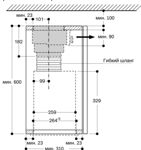
Разрез навесного шкафа с AC 200 и AA 211 812
