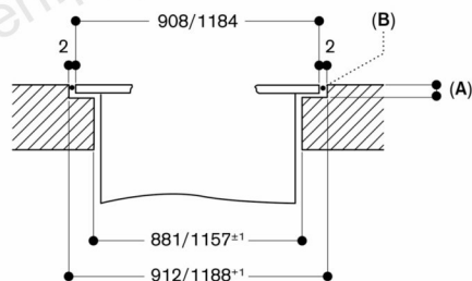
Δ: 3.5 0.5 мм B: заполнить силиконом
