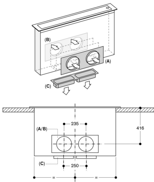
A: Подключение спереди с AD 754 049. B: Подключение сзади с AD 754 049. C: Подключение снизу с AD 854 050. Размеры в мм.
