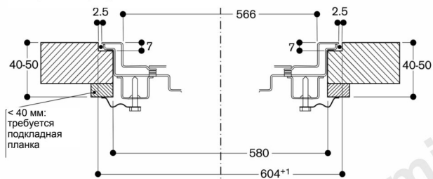
Поперечный разрез
