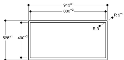
Вид сверху
