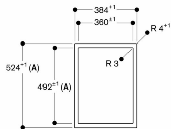
Вид сверху
